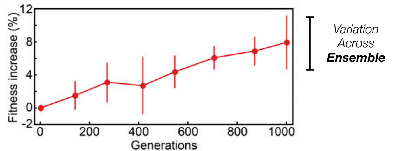
Lang et al ( Genetics , 2011)
